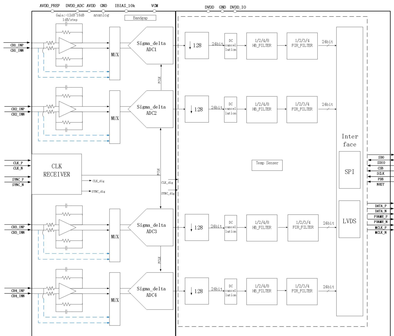
图 1 CX74E0/CX74E0N 功能框图
