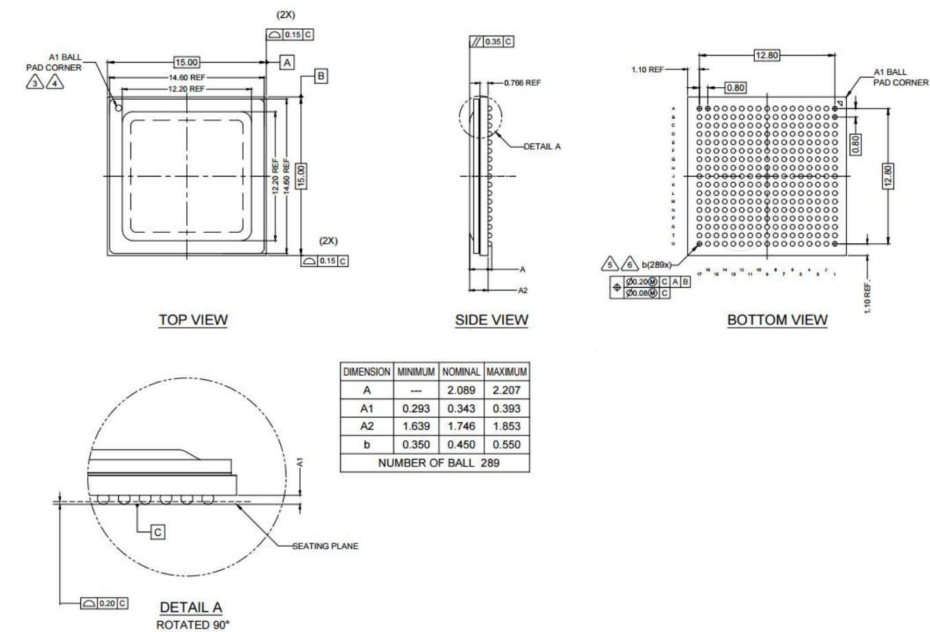
图 3 封装尺寸图
