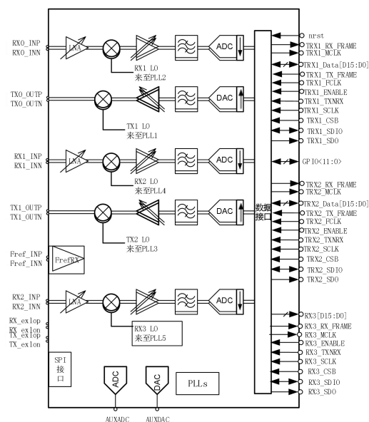
图 1 器件功能框图
