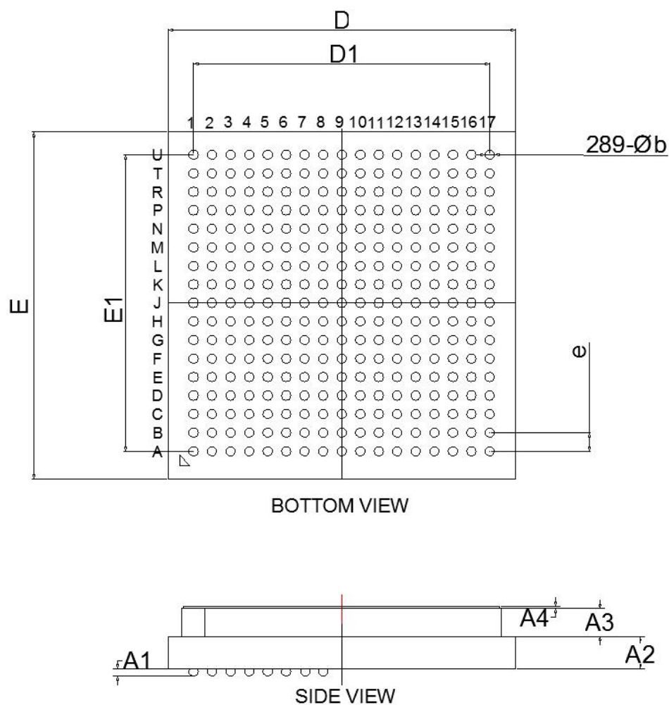
图 57 封装尺寸图
